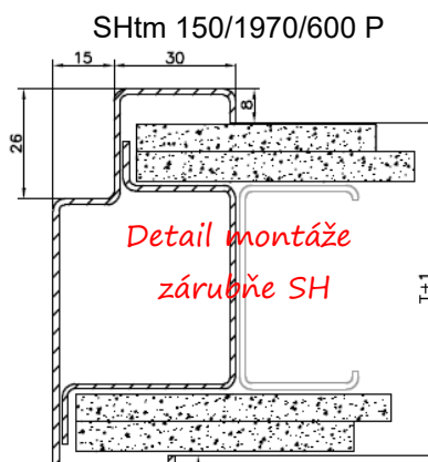
Detail montáže zárubne SH
