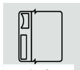
Detail protiplechu - otvor pre strelku a závoru
